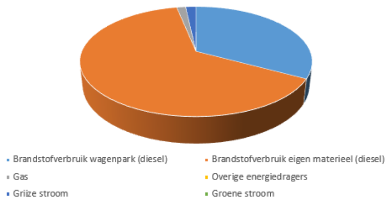
CO2 Footprint
